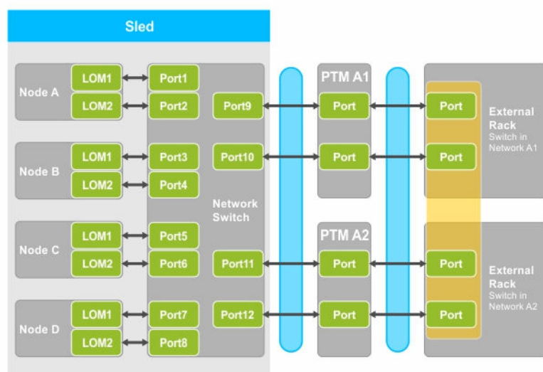
Abbildung 5. Standard-Konfiguration
