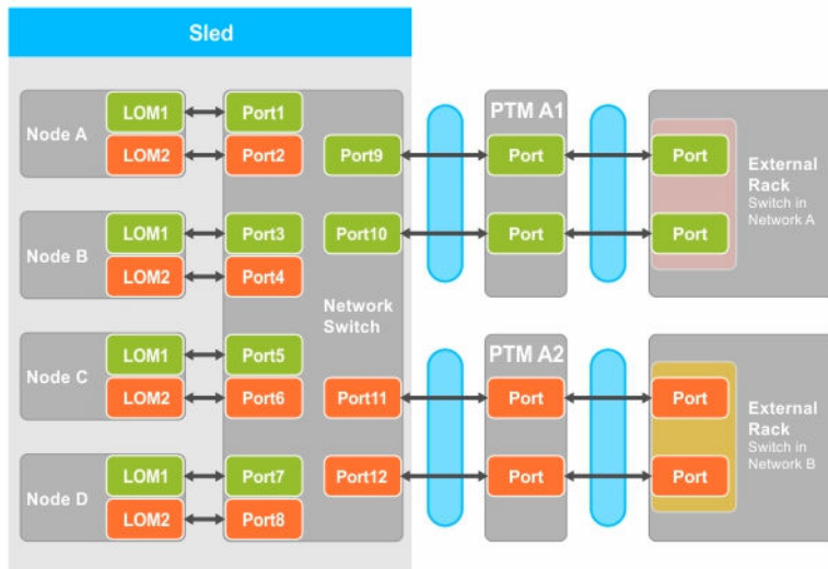
Abbildung 7. Isolierte Netzwerk-Konfiguration
